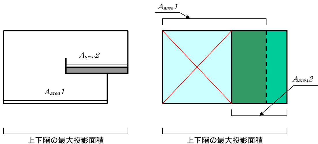
断面図
